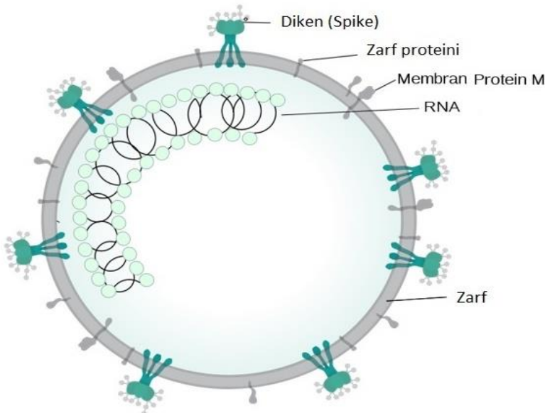
A-Covid-19 virüsü şematik yapısı
